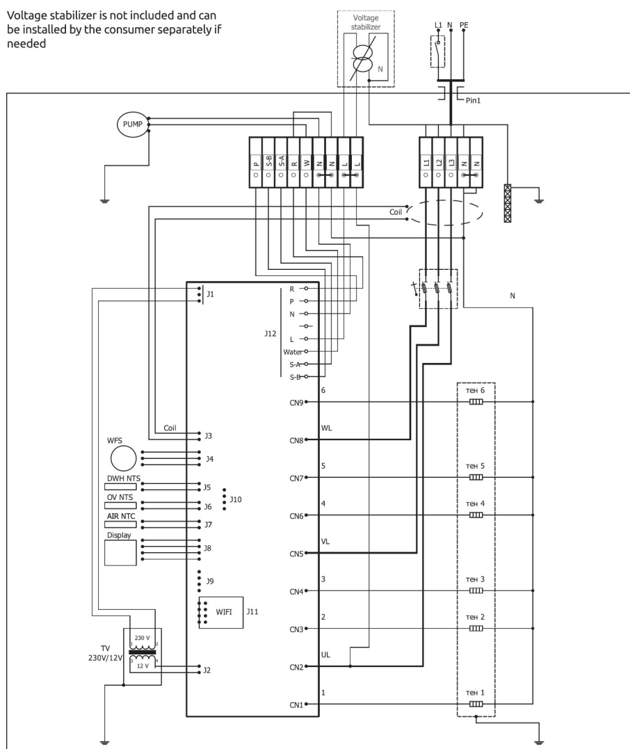
Εικόνα 14 – Σχέδιο σύνδεσης των λεβήτων ESPRO 4,5 kW, 6 kW και 7,5 kW σε μονοφασικό δίκτυο 230V (50Hz).
