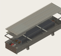
PB ΧΩΡΙΣ ΑΝΕΜΙΣΤΗΡΑ Φυσική συναγωγή, χωρίς ρεύμα.
